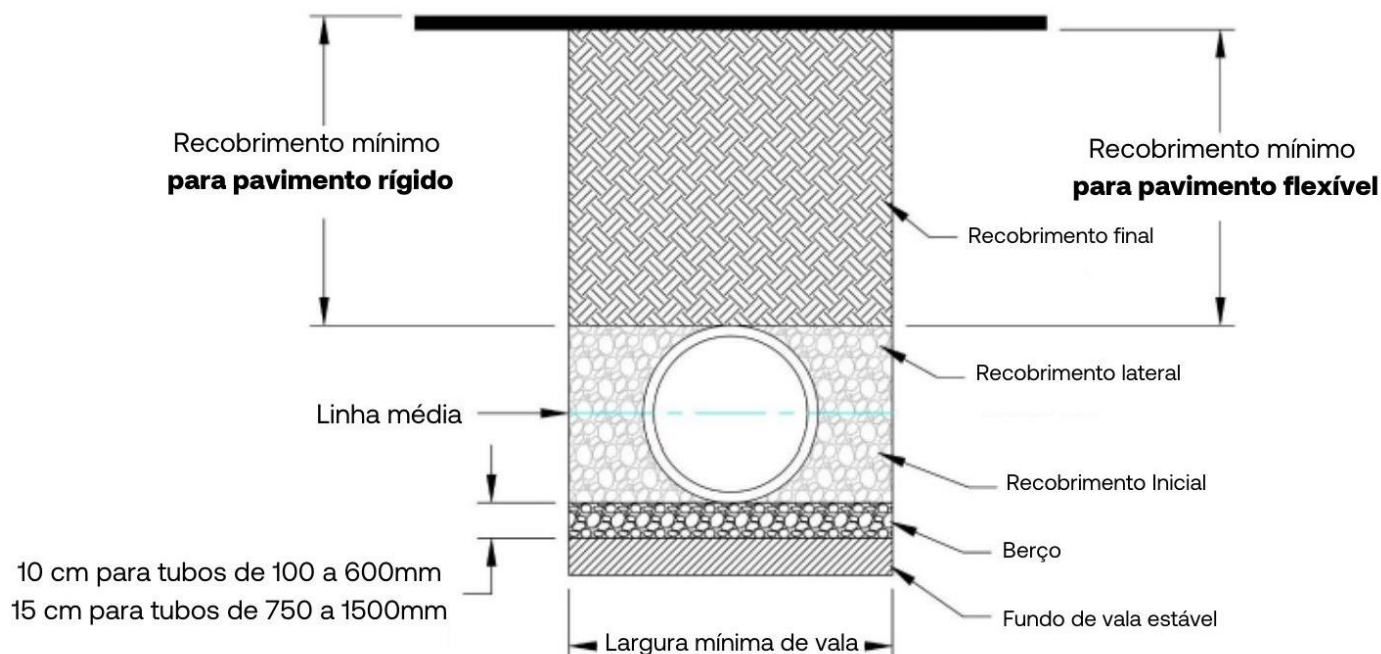
Figura 1 – Sessão Típica de instalação de Tubulações SaniPro ADS Tigre
